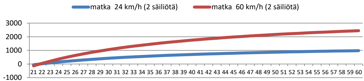
Bild 4 Största avståndet till släckvattenstationen från olycksplatsen i förhållande till vattenstationens vattenkapacitet
